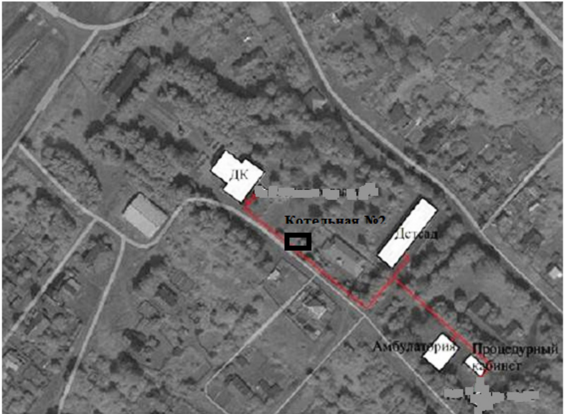
Схема теплосети котельной №2 пос. Космынино
